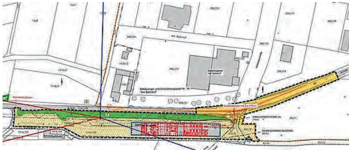
Lageplan 1 zur Aufstellung des vorhabenbezogenen Bebauungs- und Grünordnungsplanes Nr. 58 „Am Bahnhof IV“ mit Teiländerung des Bebauungsplanes Nr. 19 „Am Bahnhof“ – Überlappungsbereich
