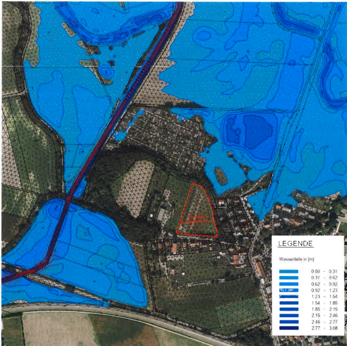
Abb. 6 Auszug aus 2D-hydraulische Berechnung, Wassertiefen des Überschwemmungsgebiets der Brautlach bei HQ100, Quelle: IB Goldbrunner, 05.04.2019
