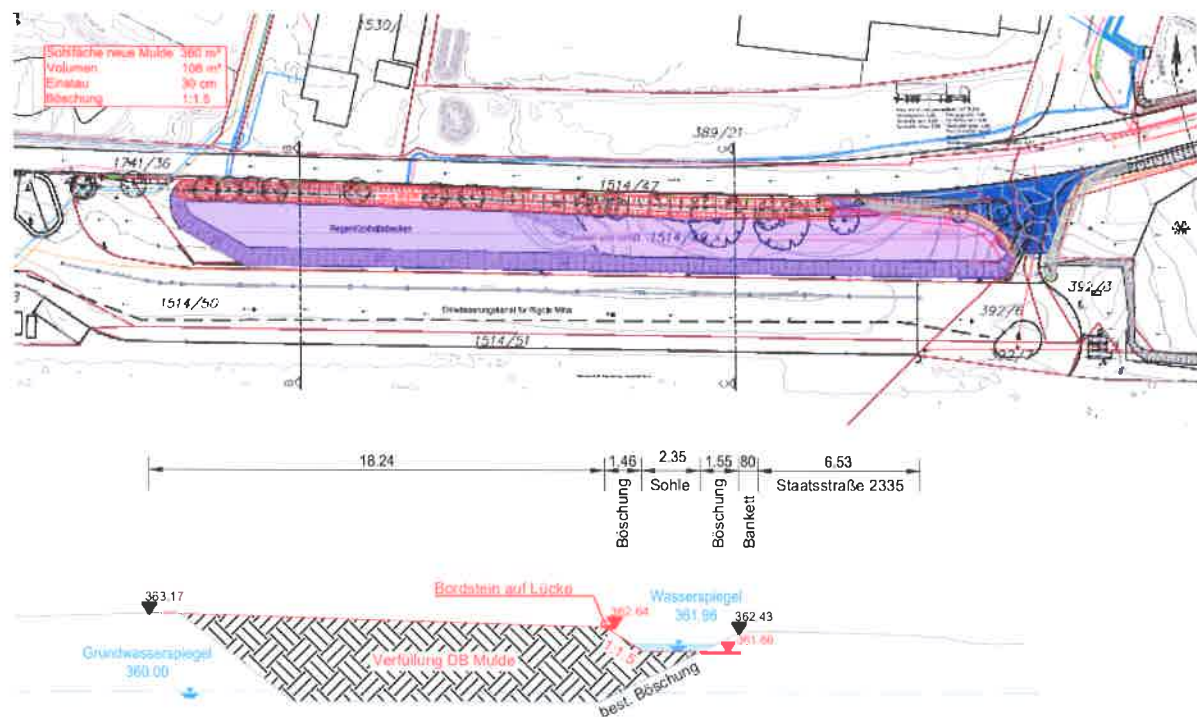
Abb. 9. Lageplan und Schnitt der neuen Mulde entlang St 2335 gem. Wasserrechtsantrag vom 03.04.2023
